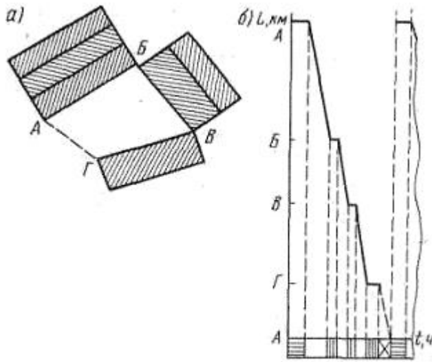
Рис. 4 – Графік роботи на розвізному маршруті При роботі на кільцевих маршрутах кількість необхідного рухомого складу:
