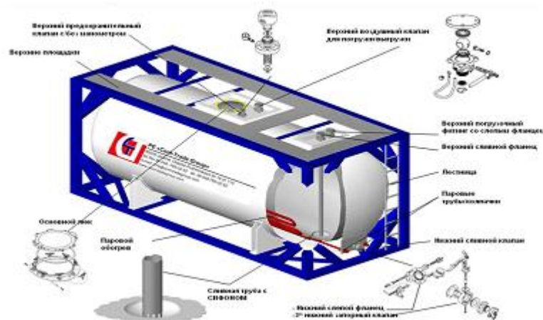
Рис. 3 – Танк-контейнер
