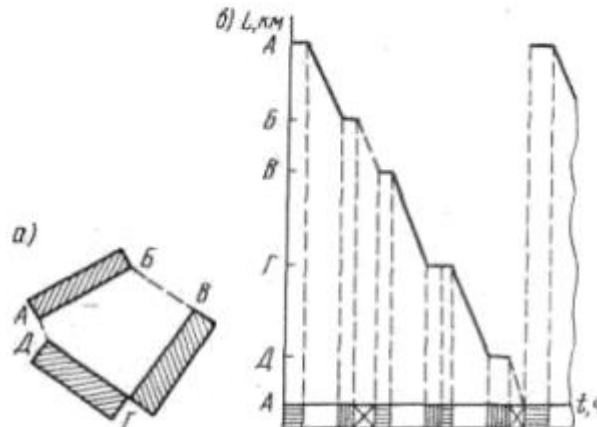
Рис. 3 – Графік роботи на кільцевому маршруті Середній коефіцієнт статичного використання вантажопідйомності за оберт
