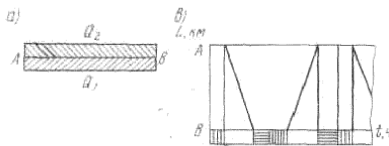
Рис.2 – Маятниковий маршрут з навантаженим пробігом в обох напрямках Час обертів рухомого складу:
